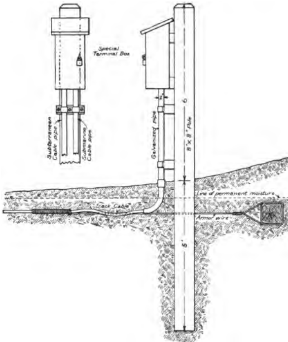
FIG. 129.—Cable box.
